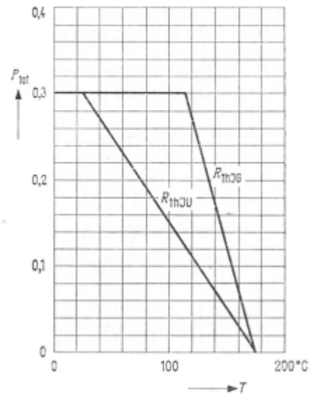
Temperaturabhängigkeit der zulässigen Gesamtverlustleistung P_{tot} = f(T) ; R_{th} = Parameter BC 177, BC 178, BC 179
