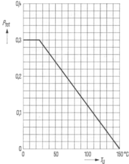
Temperaturabhängigkeit der zulässigen Gesamtverlustleistung P_{tot} = f(T_U) BC 157, BC 158, BC 159 BC 257, BC 258, BC 259
