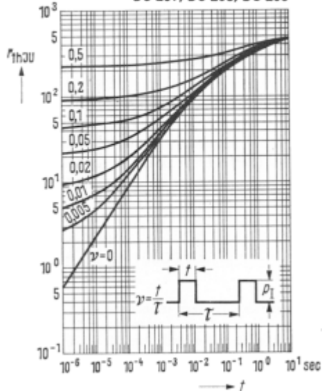
Zulässige Impulsbelastbarkeit r_{thJU} = f(t) BC 157, BC 158, BC 159 BC 257, BC 258, BC 259
