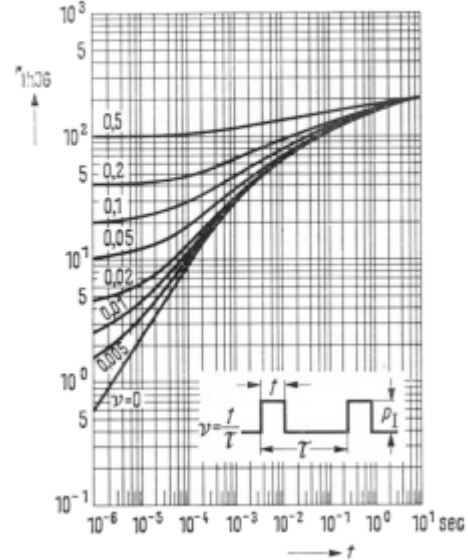
Zulässige Impulsbelastbarkeit r_{thJG} = f(t) BC 177, BC 178, BC 179
