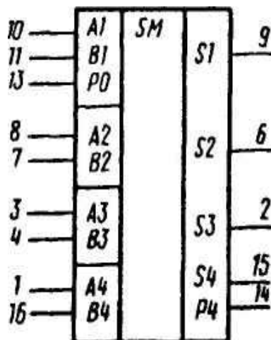
Условное графическое обозначение К155ИМЗ, КМ155ИМЗ
