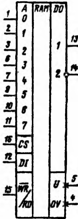
Условное графическое обозначение K176PY2
