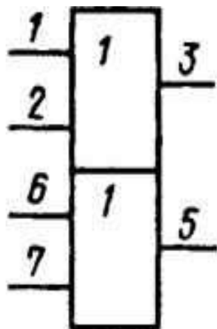
Условное графическое обозначение К155ЛЛ2
